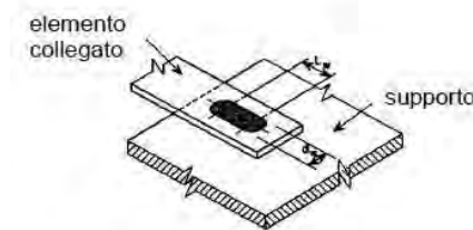
Figura C4.2.36 –Saldature oblunghie a bottone
