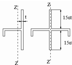
Figura C4.2.12 - Irrigidimenti longitudinali dei pannelli d'anima
