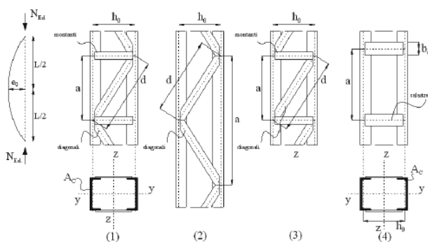
Figura C4.2.7-Aste composte costituite da due correnti uguali
